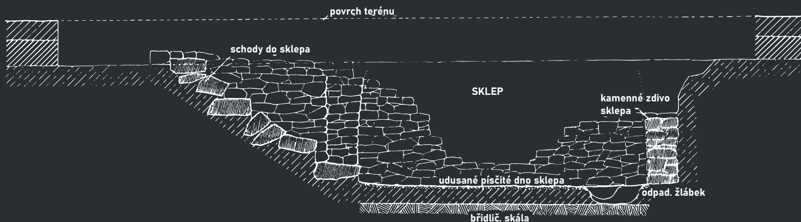
ŘEZ I–J
